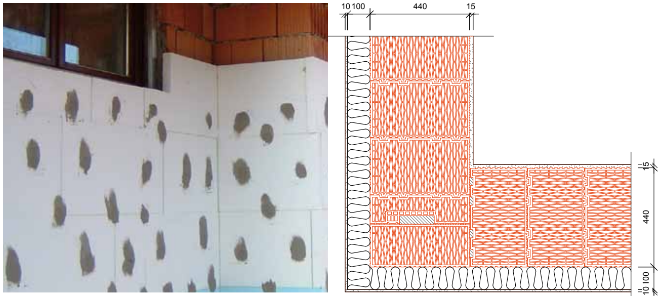
Řešení obvodového zdiva cihelného pasivního domu HELUZ HIT - HELUZ THERMO STI 44 + 100 mm izolace
